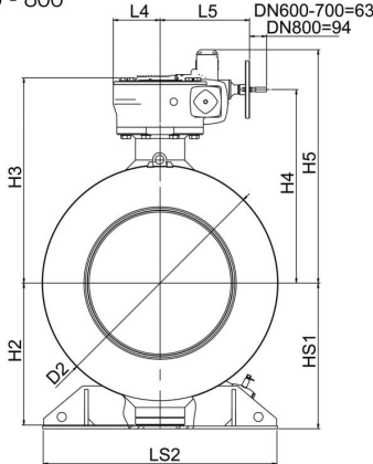
DN 600 - 800
